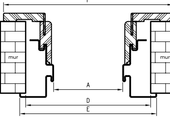
Profil ościeżnicy
