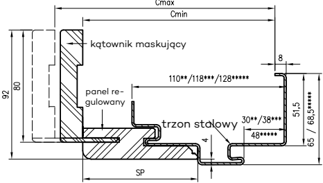
Profil ościeżnicy
